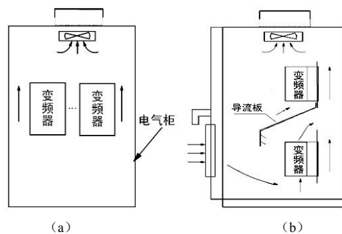
图 3-2 多台变频器的安装
