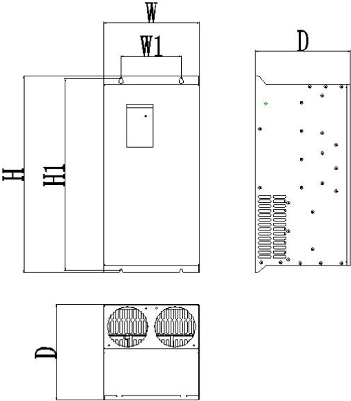
图 2-3 C500 中压矢量变频器标准外形尺寸(适用于 45~110kW 机型)
