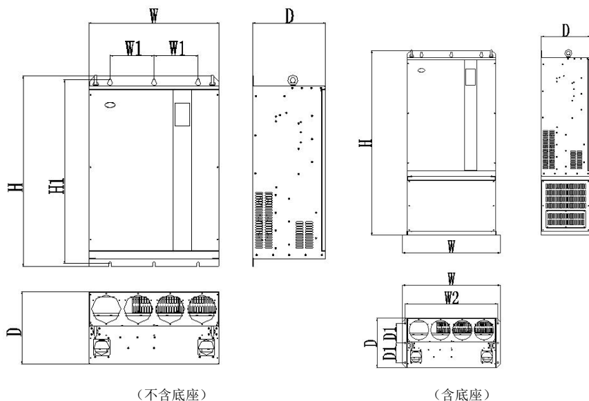
图 2-4 C500 中压矢量变频器标准外形尺寸(适用于 132~1000kW 机型)
