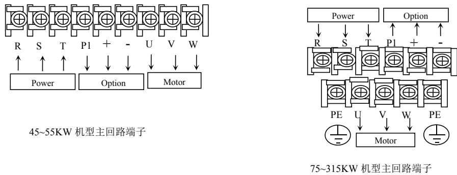
图 3-5 C500 系列主回路接线端子图
